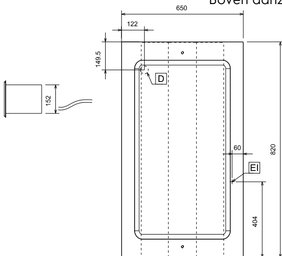
Boven aanzicht
