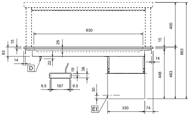
Zij aanzicht
